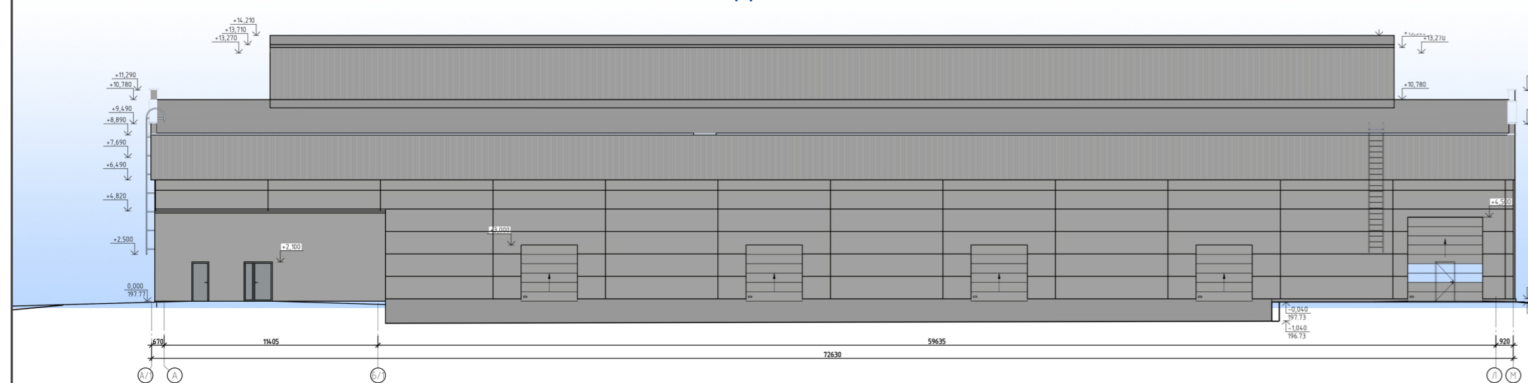
Фасад А-М
